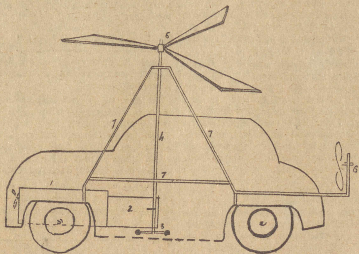
Tak wygląda auto-pter, samochód latający, według opatentowanego w Szkocji wynalazku polskiego: 1) silnik z kompresorem, 2) skrzynka biegów, 3) żyroskop, 4) oś napędowa rotora (wiatrak), 5) rotor, 6) śmigło pomocnicze, 7) rama składana.
