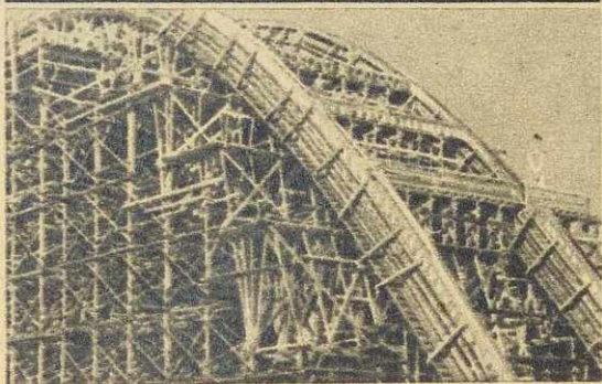
To nie kolejka górską w wesołym miasteczku. To olbrzymia hala sportowa, która powstaje w Łodzi. Na zdjęciu montaż jednego z łuków. Na rusztowania zużyto drzewa z 25 ha lasu
