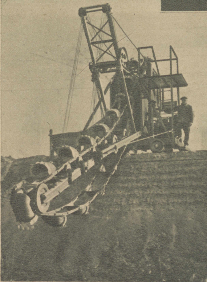
Współzawodnictwo, organizacja i mechanizacja pracy, to trzy czynniki, decydujące o szybkiej odbudowie kraju. Na zdjęciu: kopaczka kubelkowa do czepiania gliny, stosowana w cegielni „Henryków” k. Słonia
