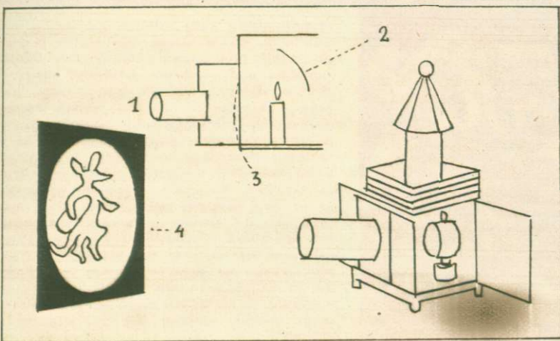
Latarnia magiczna: 1. obiektyw, 2. reflektor, 3. kondensator, 4. ekran.
