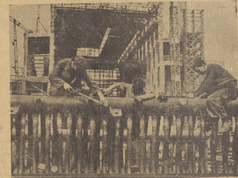
Prace przy budowie wielkiej siłowni „Jaworzna II” postępują szybko naprzód. Już w początkach przyszłego roku ruszy pierwszy turboszpół. Montaż turbiny, dostarczonej przez ZSRR, odbywa się pod kierownictwem inżynierów radzieckich.
