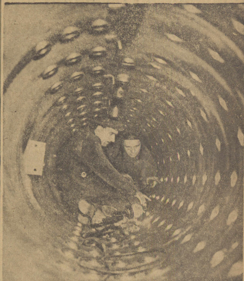
Za kilkanaście dni gotów będzie pierwszy kotłowni w elektrociepłowni „Żerania” w Warszawie, rozpoczną się wtedy próby techniczne. „Żerania” — z pierwszego bloku energetycznego — da prąd już w lipcu bież. roku. Na zdjęciu: fragment montażu tzw. walczaka węglowego — w bębnie pracują monterzy Marian Kościak i Jan Nawrot.
