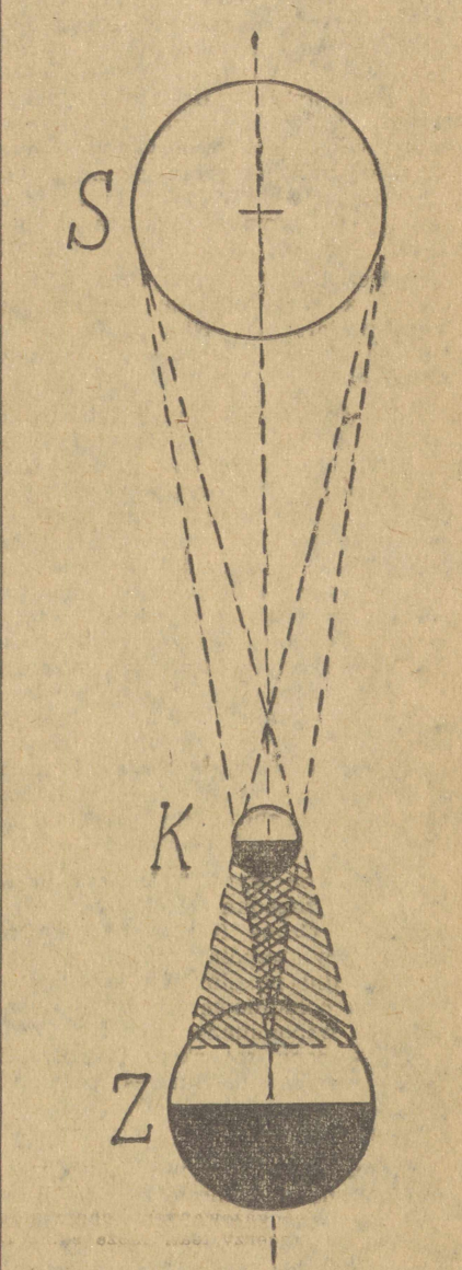
Schemat zaćmienia Słońca: S — Słońce, Z — Ziemia, K — Księżyc.
