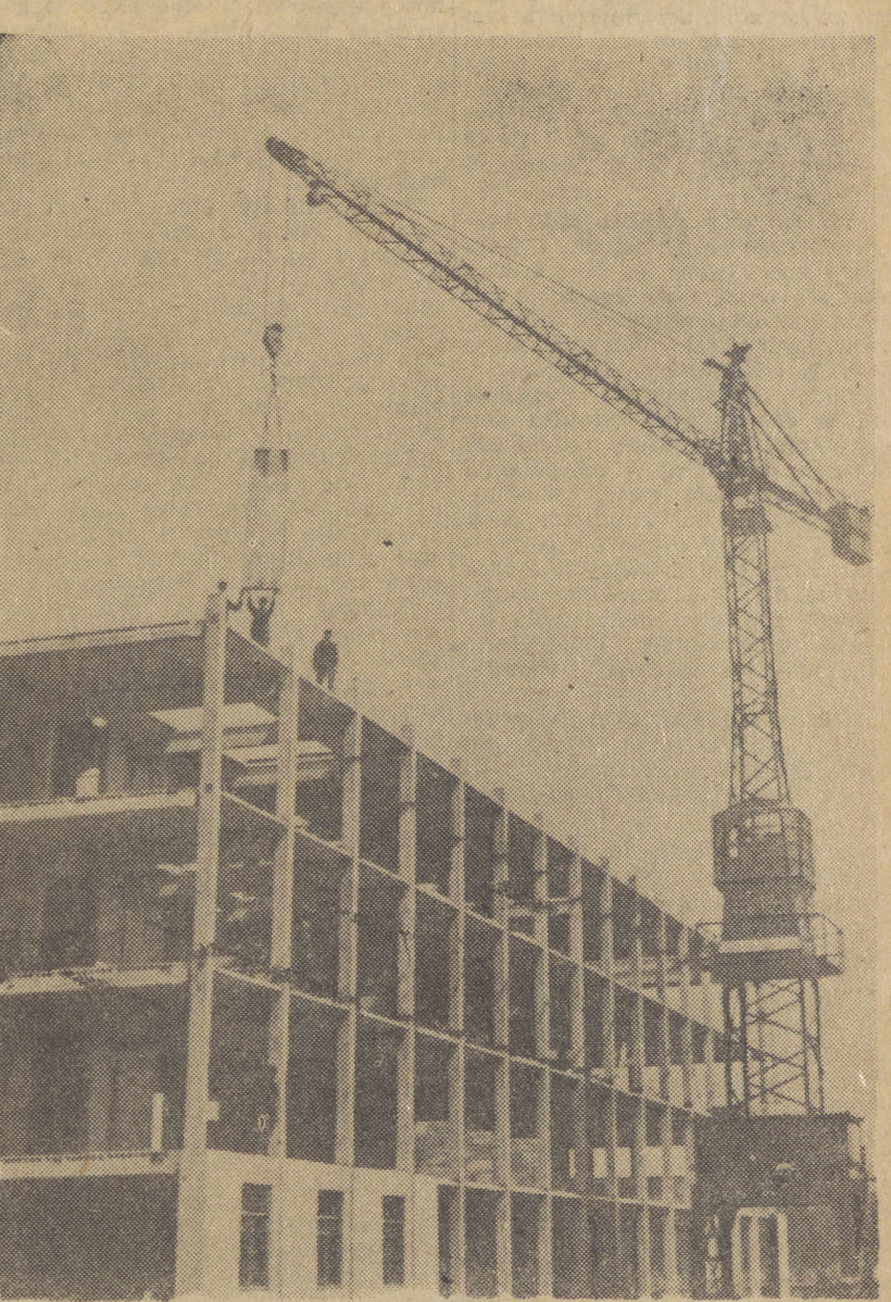
W osiedlu Jasinowackiej fabryki maszyn górniczych (obwód Stalowski) montuje się pierwszy dom mieszkalny z dużych płyt. Na zdjęciu: montaż ścian 4 piętra.
