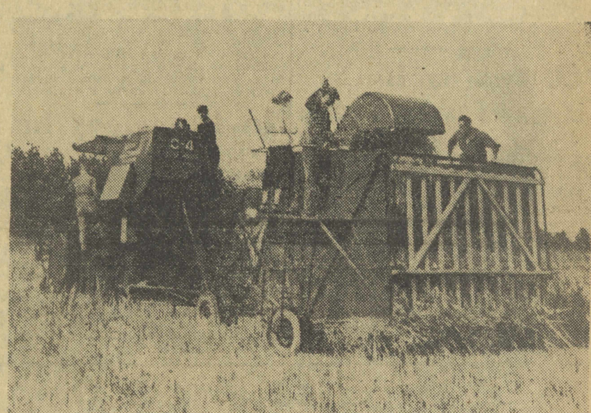
Sprzęt zboża przy pomocy kombajnu produkcyjnego radzieckiego w PGR — Izmanowice (pow. Żółtyja). Przy pracach żniwnych pomagają studenci Wyższej Szkoły Rolniczej w Krakowie, przebywający w gospodarstwie na praktykach. CAF fot. Data
