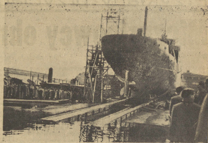
W stoczni szczecińskiej wodowano kadłub nowego rudowęglowca, którego nadano nazwę S/S „Malbork”. Budowa nowego kadłuba zakończona została w czasie o 60 proc. krótszym niż budowa pierwszego kadłuba w tej samej stoczni. Na zdjęciu: S/S „Malbork” na pochylni na chwilę przed wodowaniem. CAF — fot. Podolski
