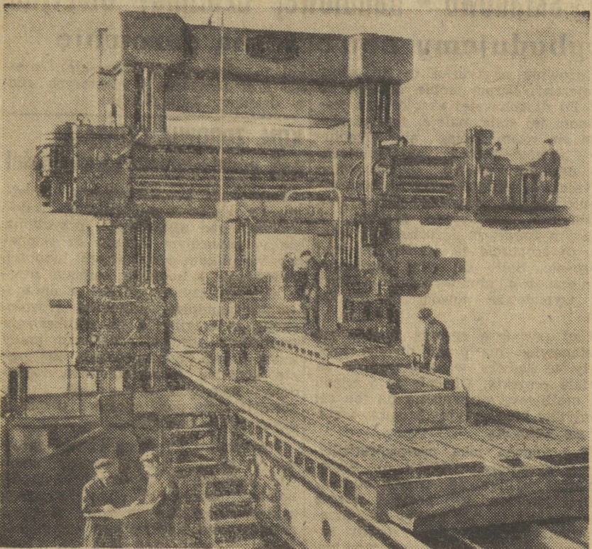
Jedyna na świecie heblarka do metali model 7288 F nowosyberyjskiej fabryki „Tiaistankohidropres”, na której można obrabiać części wagi do 100 ton. Pojęcie o wielkości obrabianych części daje stojąca na niej zwykła heblarka, a obok niej — ludzie. Zdjęcie tej heblarki zamieścił tygodnik Sowietiskij Sojuz jako ilustrację do artykułu „Technika piątej pięciolatki”.
