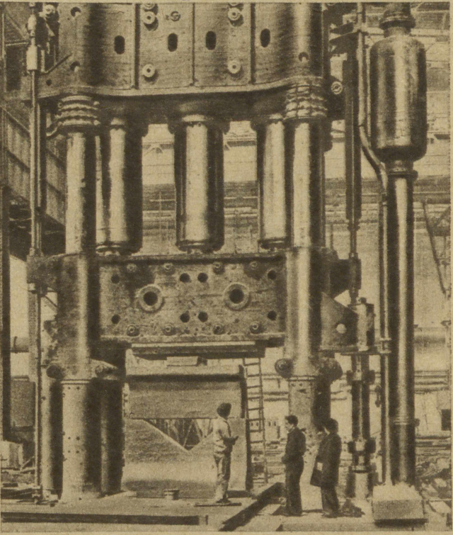
O ponad 60 proc. wzrosła produkcja niemieckiego przemysłu w ciągu ub. 4 lat. Oto np. olbrzymia 6000-tonowa prasa, dzieło niemieckich inżynierów wmontowana niedawno w jednym z zakładów metalowych NRD.
