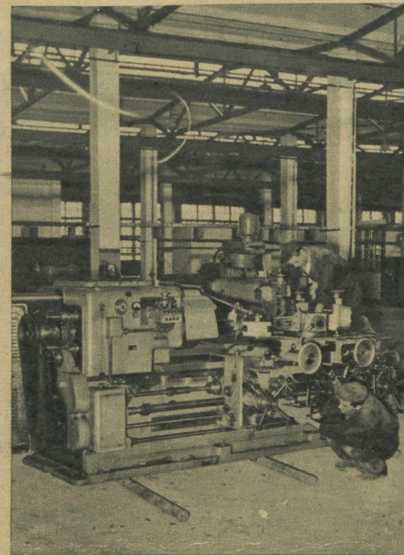
W szybkim tempie powstaje w Kielcach pierwsza w kraju fabryka wysokopiętnych armatur, budowana w oparciu o dokumentację techniczną i dostawy maszyn z ZSRR. Oto fragment hali mechanicznej, w której brygada Jana Malinowskiego ustawia niedawno otrzymane maszyny.
