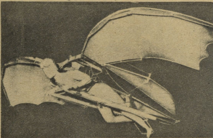
Model szybowca Leonarda da Vinci (napęd nożny).
