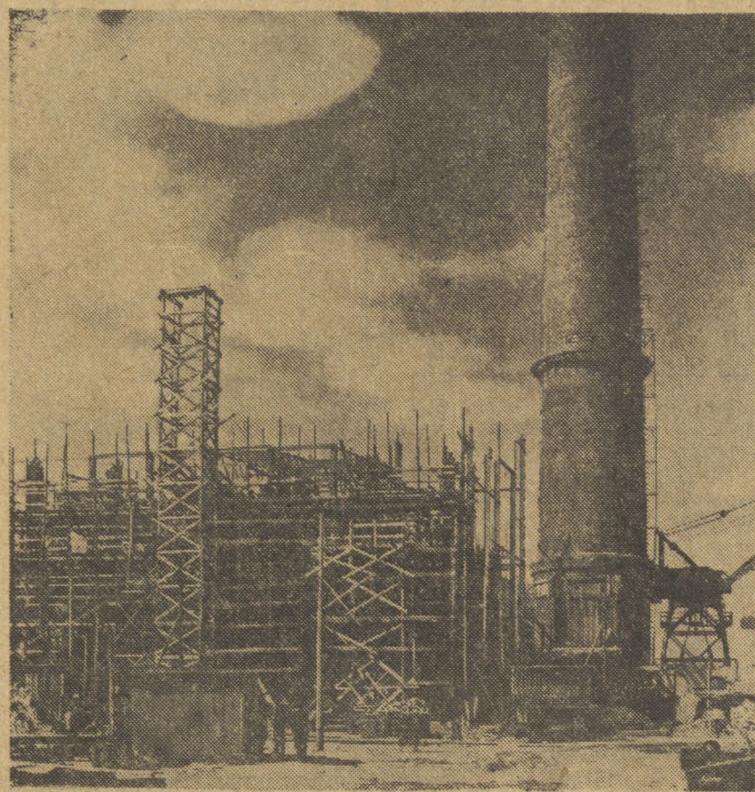
1 maja ruszy olbrzymia cementownia w Wierzbicy — jeden z wielkich zakładów przemysłowych Planu Sześcioletniego. W czasie przeprowadzania końcowych prac wiele szkieletów i betoniarzy przekracza dwukrotnie normy produkcyjne. Na zdjęciu fragment budowy.
