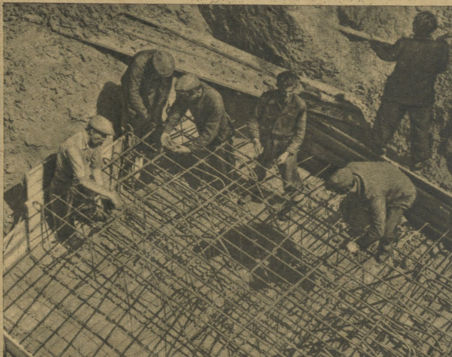
Prace dobiegają końca. Wkrótce już cementownia-gigant w Wierzbicy, wielka inwestycja planu 6-letniego, podejmie produkcję. Brygada monterska Romana Dziadkiewicza z „Mostostalu” „finiszuje” wyrabiając 180 proc. normy (zdjęcie po lewej). Na innym „odcinku” kończą pracę przodujący zbrojarze z brygady Skawińskiego. Płatanina żelaznych prętów pokryje się wkrótce betonem.
