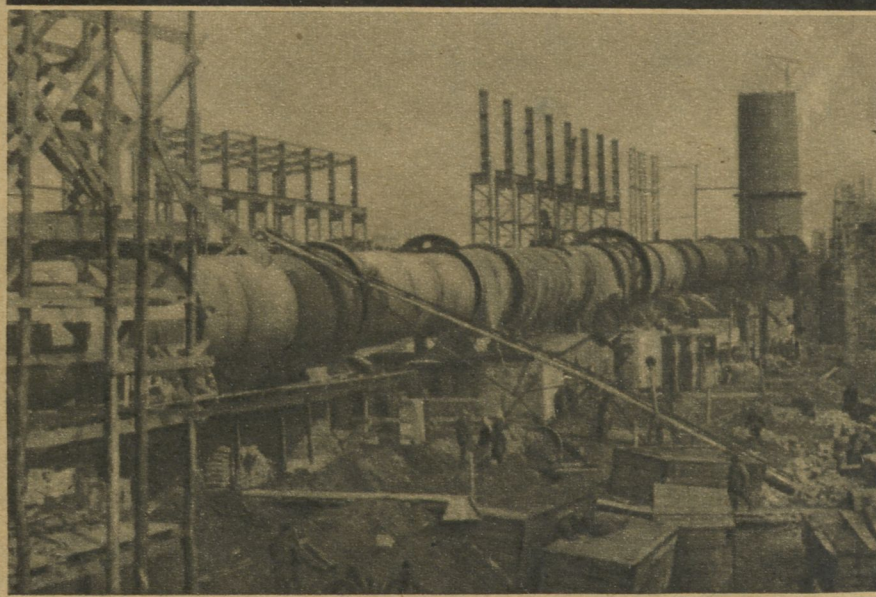
Wzdłuż potężnego pieca obrotowego rozciąga się jeszcze rumowisko cegieł i czę- ści budulca. Ale uporządkowanie terenu nie potrwa długo. Tu już potrzebna jest tylko końcowa „toaleta”.
