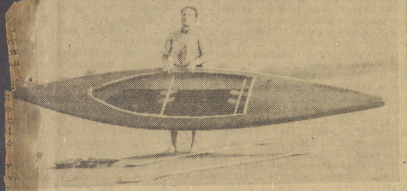
Kajak zbudowany na kleju bakelitowym, bez gwoździ i śrub.
