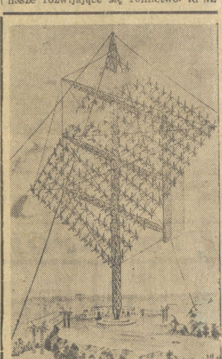
Rys. 2. Ogólny widok zaprojektowanej w ZSRR wielkiej elektrowni, poruszanej siłą wiatru.
