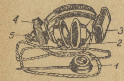
Aparat do badania pracy maszyn: 1) mikrofon z igłą, 2) słuchawki z gumowymi pierścieniami, 3) baterijka w puszcze od kieszonkowej latarki, 4) puszka z transformatorem, 5) wtycznik.
