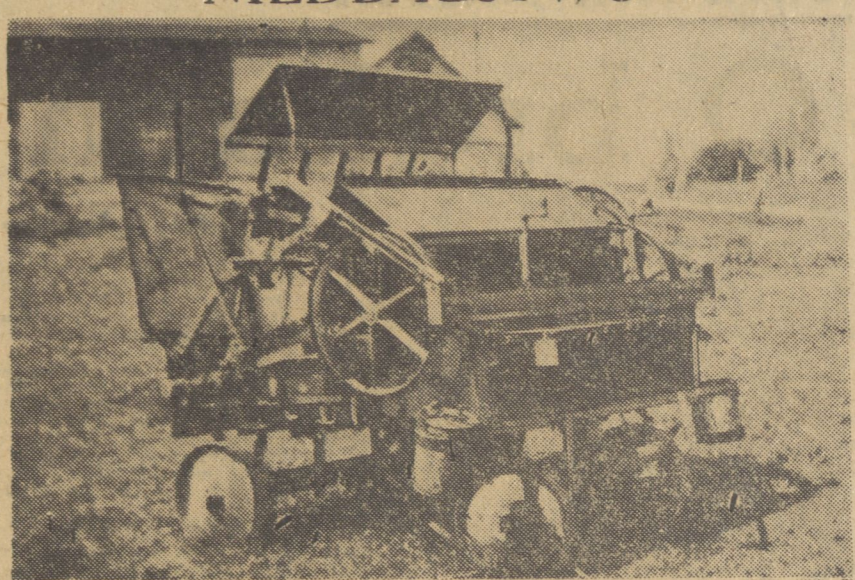
Ta prasa do słomy stoi już od dłuższego czasu bez opieki w okolicy spółdzielni produkcyjnej Wszakajty pow. Górowo Hławeckie. Maszyna niebezpieczna, choć znalazłaby niewątpliwie zastosowanie w spółdzielni, lub okolicznych PGR.
