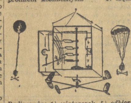
Radiosonda: 1) wiatraczek, 5) odbiornik, 6) źródło prądu, 7) nadajnik radiowy.
