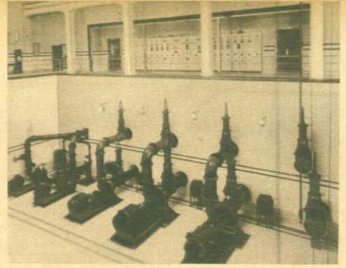
Hala pomp w Zakładzie Filtrów Pośpiesznych.
