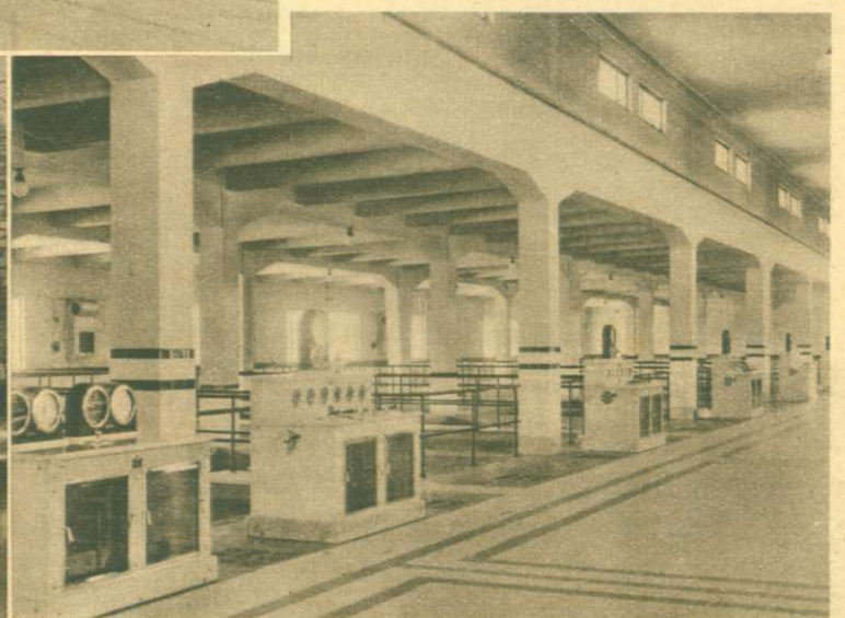
Hala filtrów pośpiesznych.
