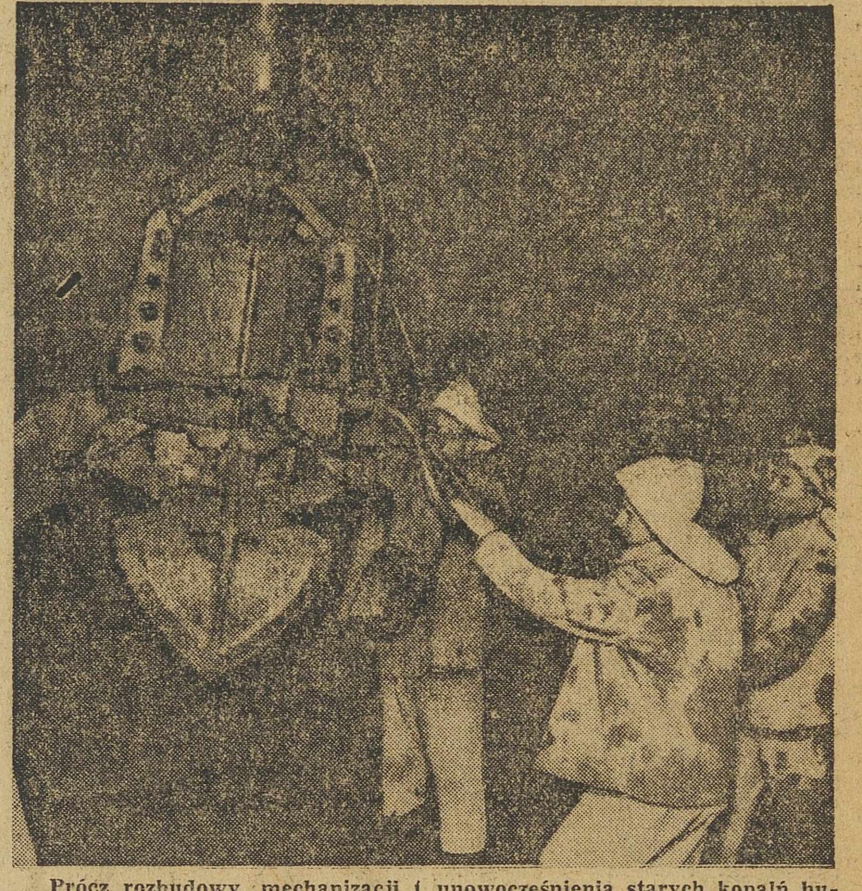
Prócz rozbudowy, mechanizacji i unowocześnienia starych kopalni budujemy także nowe. Na zdjęciu: budowa kopalni węgla, najnowocześniejszymi metodami radzieckimi i sprzętem dostarczanym przez ZSRR. Ładowarka (czepak szczytowy) — przy pracy. Wydobyt kamień przenosi kibel do góry a jednocześnie służy obmurowaniu ściany. Foto AR.
