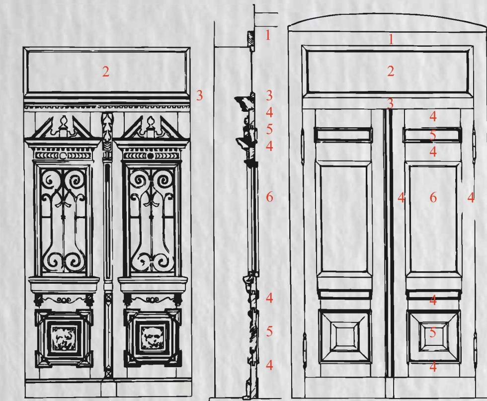
Schemat konstrukcji drzwi ramowo-płycinowych z poszczególnymi elementami
